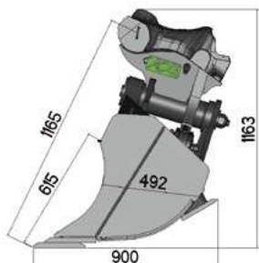
Profil 5CP1E 2 x 45° - 2 Vérins
